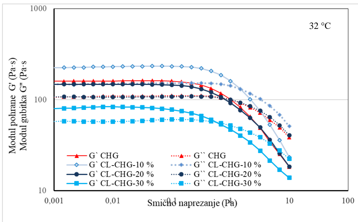
Slika 17. Grafički prikaz ovisnosti modula gubitka G'' i modula pohrane G' o smičnom naprezanju za izvorni CHG i CL-CHG liposomski gel pri 32 °C.
