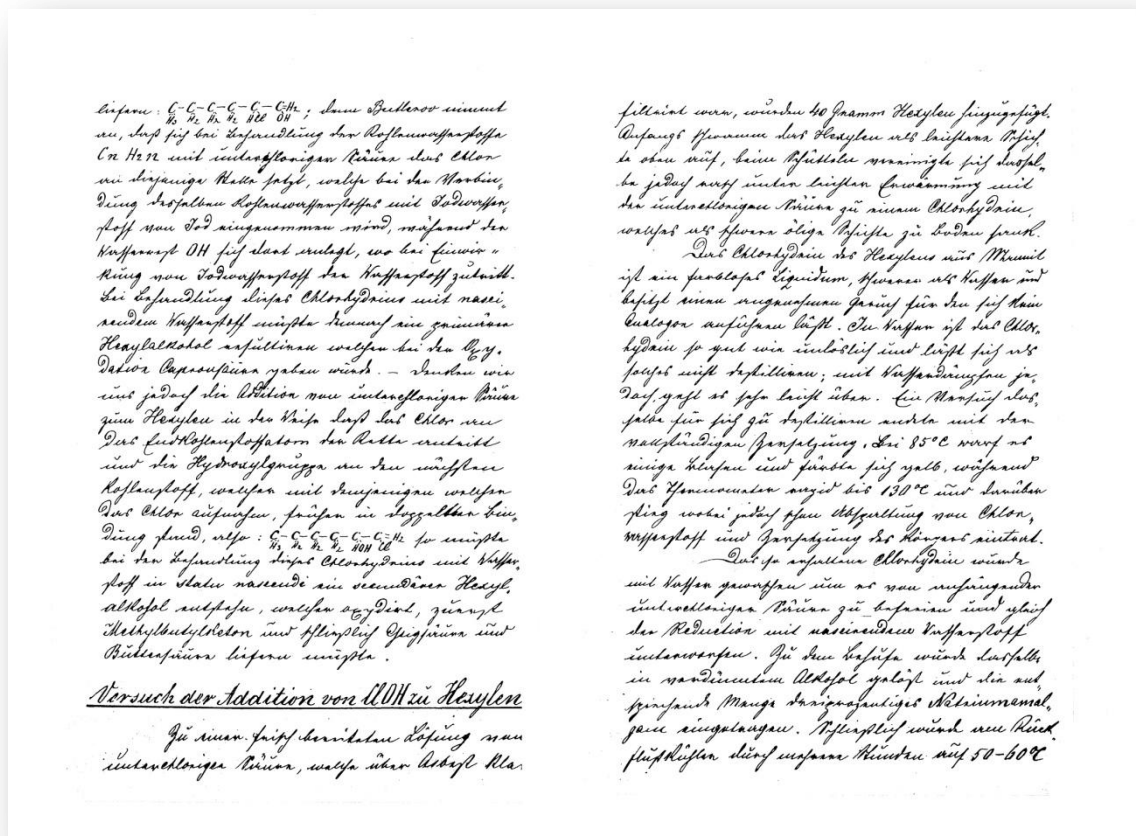
Slika 48 Dio Domčevog doktorskog rada u kojem je opisana adicijska reakcija HClO na heksen (Knjižnica GRAZ)
