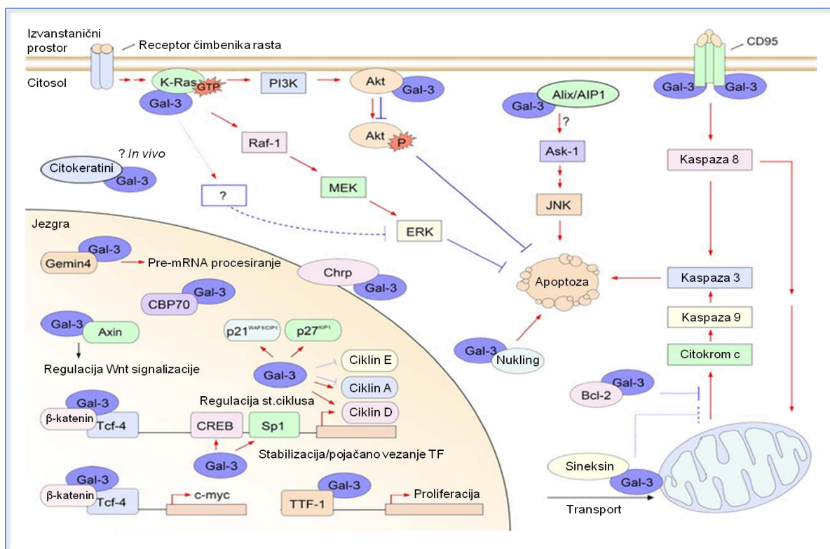
Slika 1.6 Funkcije galektina-3 unutar stanice. Crvene strijelice označuju pozitivne, a plave negativne učinke. Akt – serinska/treoninska kinaza Atkt, Ask-1 (eng. apoptosis signal-regulating kinase 1) – kinaza koja upravlja apoptoznom signalizacijom 1, CBP70 (eng. carbohydrate binding protein 70) – protein koji veže ugljikohidrate 70, Chrp (eng. cysteine- and histidine-rich protein) – protein bogat cisteinom i histidinom, CREB (eng. cAMP-response-element-binding protein) – protein koji veže cAMP-response-element, ERK (eng. extracellular signal-regulated kinase) – kinaza regulirana izvanstaničnim signalom, Gal-3 – galektin-3, GTP (eng. guanosine triphosphate) – gvanozin trifosfat, JNK – c-Jun NH 2 -terminalna kinaza, MEK – mitogenom aktivirana protein/ERK kinaza, P – fosfat, PI3K (eng. phosphatidylinositol 3-kinase) – fosfatidil-inozitol 3 kinaza, Raf-1 – serinska/treoninska kinaza Raf-1, Tcf-4 (eng. T-cell factor 4) – faktor limfocita T 4, TF (eng. transcription factor) – transkripcijski faktor, TTF-1 (eng. thyroid-specific transcription factor) – transkripcijski faktor specifičan za štitnjaču. Preuzeto i prilagođeno iz [58].
