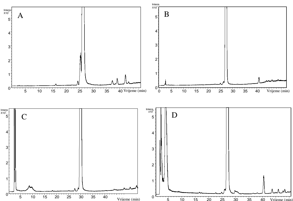
Slika 29. TIC kromatogrami aktivnih ljekovitih tvari (1 000 µg/mL), Uzorak 1 (A) i Uzorak 2 (B) te gotovih ljekovitih oblika atorvastatina, Uzorak 1 (C) i Uzorak 2 (D).
