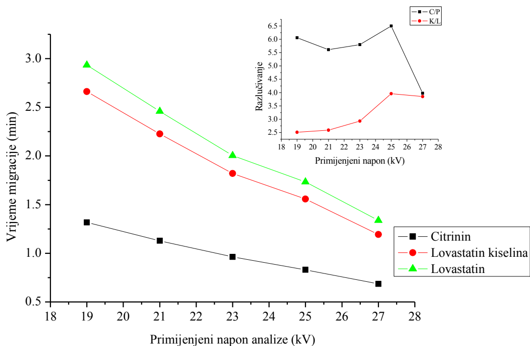
Slika 43. Ovisnost vremena migracije o primijenjenom naponu analize. Umetak slici: Ovisnost razlučivanja između analita o primijenjenom naponu analize.
