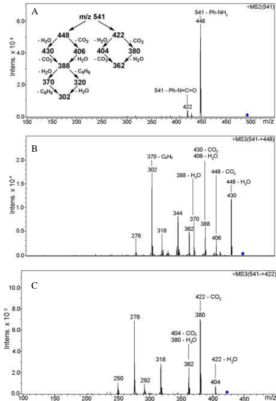
Slika 27. ESI-MS 2 spektar molekuskog iona m/z 541 laktona atorvastatina (A), ESI-MS 3 spektri fragmentnih iona m/z 541 → 448 (B) i m/z 541 → 422 (C) desfluoroatorvastatina te predložena fragmentacijska shema.
