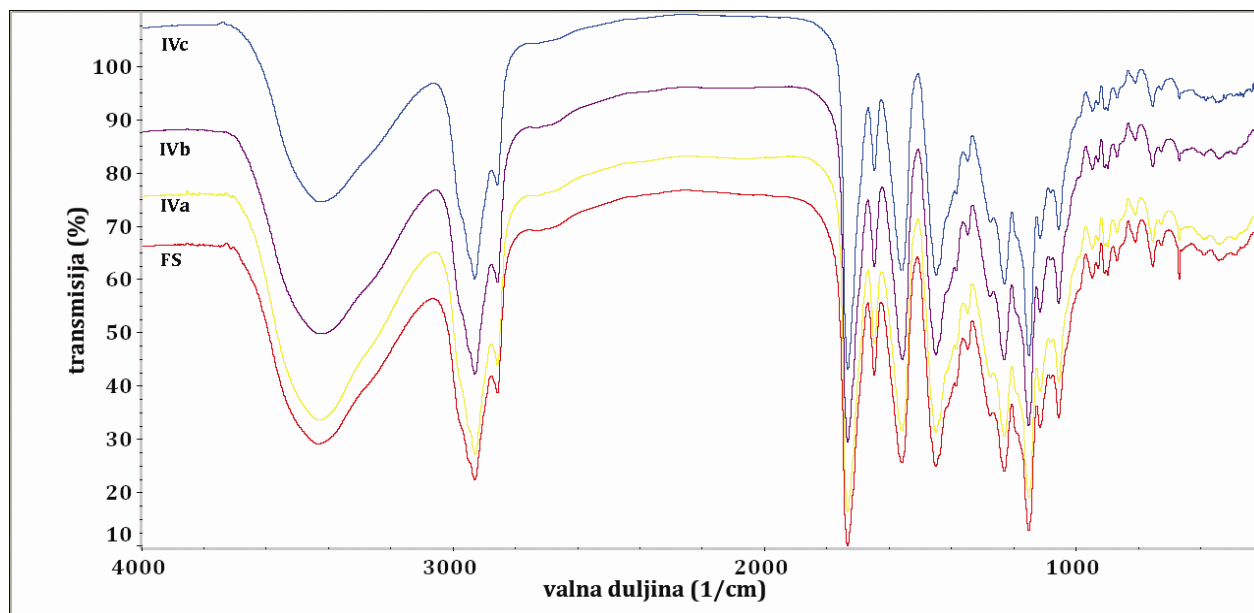
Slika 5 - 21. FTIR spektri mikročestica s omjerom lijeka i polimera 2 : 1 ( m/m ) sušenih raspršivanjem iz a) metanola; b) metanol-etanolske smjese (50 : 50, m/m ) i c) aceton-izopropanske smjese (40 : 60, m/m ) u usporedbi s fizičkim smjesama (FS) lijeka i polimera
