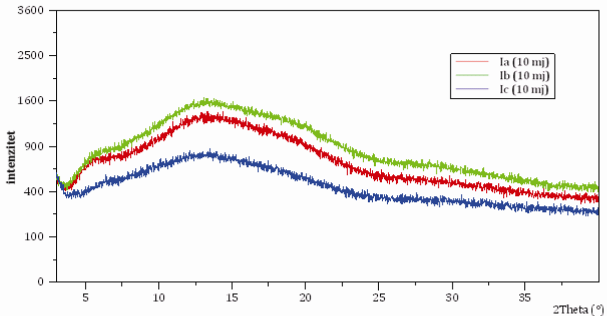
Slika 5 - 24. Difraktogram mikročestica s omjerom lijeka i polimera 1 : 5 ( m/m ) sušenih raspršivanjem iz a) metanola; b) metanol-etanolske smjese (50 : 50, m/m ) i c) aceton-izopropanolne smjese (40 : 60, m/m ) nakon deset mjeseci uskladištenja na 25 °C/60%RV
