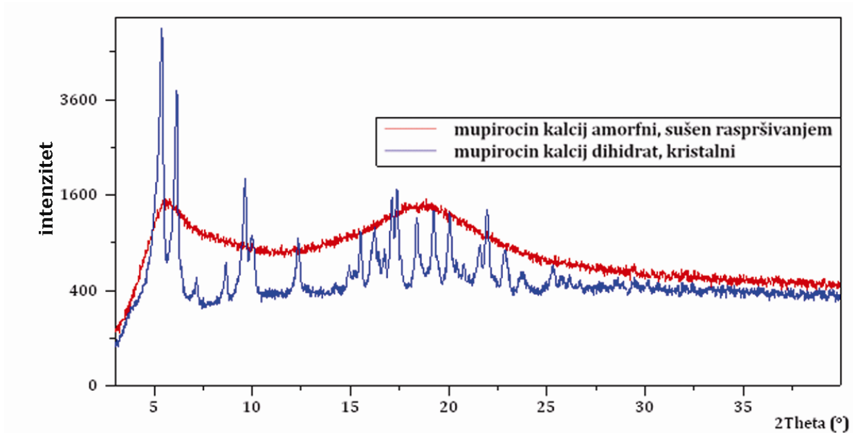
Slika 5 - 2. Difraktogram lijeka u izvornom obliku (kristalni) i onoga dobivenog sušenjem raspršivanjem (amorfni)
