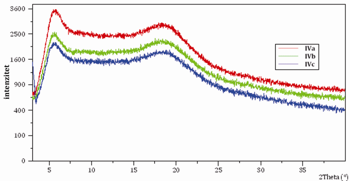
Slika 5 – 19. Diffraktogram mikročestica s omjerom lijeka i polimera 2 : 1 ( m/m ) sušenih raspršivanjem iz a) metanola; b) metanol-etanolske smjese (50 : 50, m/m ) i c) aceton-izopropanolske smjese (40 : 60, m/m )
