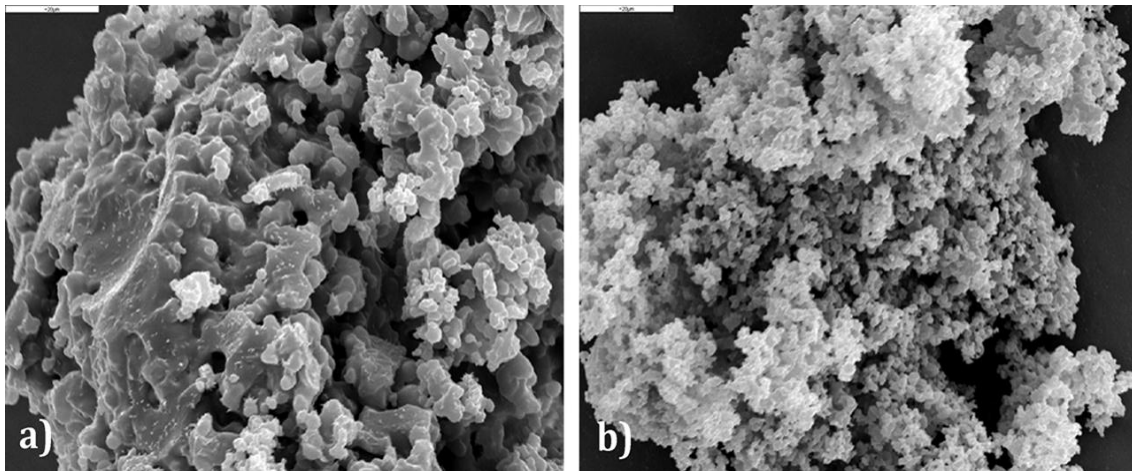
Slika 5 – 28. SEM slike mikročestica s omjerom lijeka i polimera 1 : 5 ( m/m ) (a) i 2 : 1 ( m/m ) (b) sušenih raspršivanjem iz aceton-izopropanolske smjese (polimer u otopljenom stanju) (skala označava 20 \mu m )
