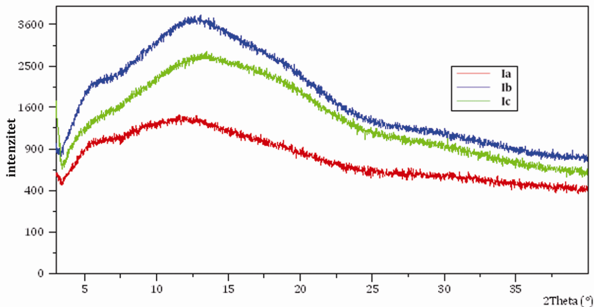
Slika 5 – 18. Diffraktogram mikročestica s omjerom lijeka i polimera 1 : 5 ( m/m ) sušenih raspršivanjem iz a) metanola; b) metanol-etanolske smjese (50 : 50, m/m ) i c) aceton-izopropanolske smjese (40 : 60, m/m )
