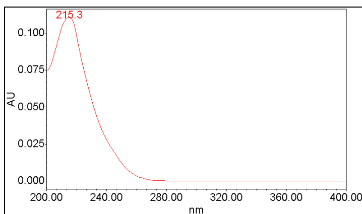
Slika 9. Apsorpcijski spektar TET, odnosno njegovih enantiomera LEV i DEX.
