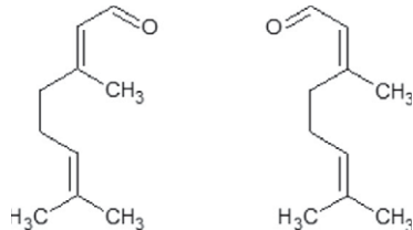
Slika 2. Strukture geraniala (lijevo) i nerala (desno)
