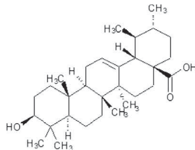
Slika 3. Struktura ursolne kiseline
