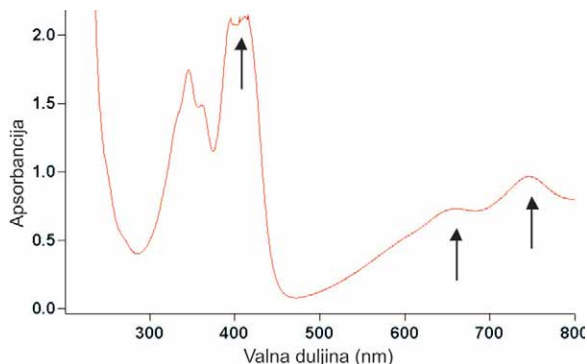
Slika 2. Spektar ABTS radikala. Apsorpcijski maksimumi nalaze se na 415, 645 i 735 nm
