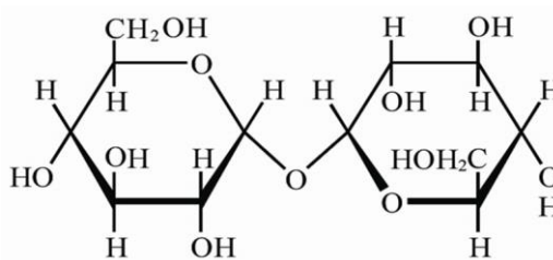
Slika 7. Trehaloza
