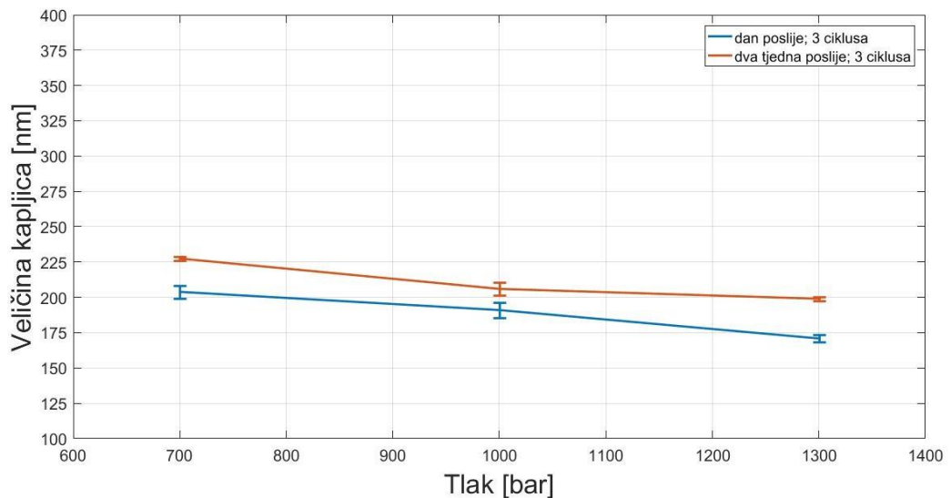
Slika 12: Utjecaj tlaka na veličinu kapljica i stabilnost nanoemulzija pripremljenih mikrofluidizacijom trima propuštanjima (3 ciklusa).
