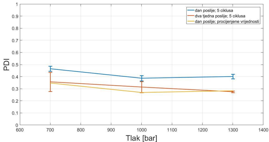
Slika 19: Utjecaj tlaka na PDI i stabilnost nanoemulzija pripravljenih metodom visokotlačne homogenizacije i pet propuštanja (5 ciklusa).
