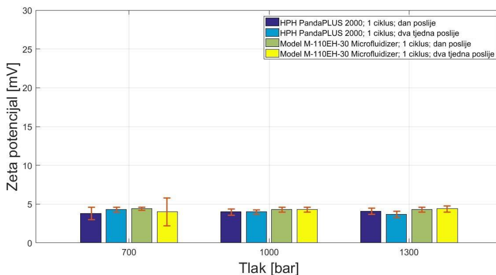
Slika 21: Utjecaj tlaka na zeta-potencijal i stabilnost nanoemulzija pripremljenih metodama visokotlačne homogenizacije i mikrofluidizacije pri jednom propuštanju (1 ciklus).
