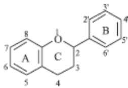
osnovna struktura flavonoida basic flavonoid structure
