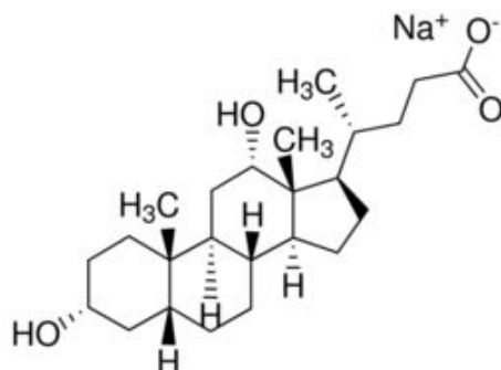
Slika 11. Na-deoksikolat ( www.sigmaldrich.com )
