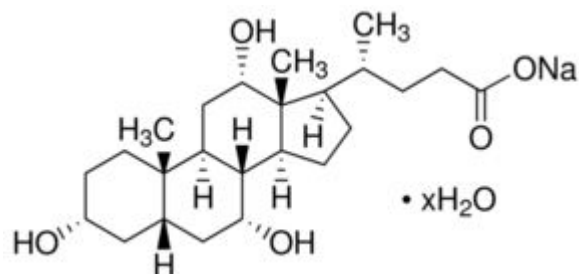
Slika 10. Na-kolat hidrat ( www.sigmaldrich.com )
