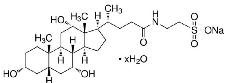
Slika 12. Na-taurokolat hidrat ( www.sigmaldrich.com )
