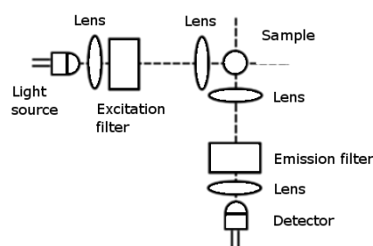
Slika 6. Shema fluorimetra
