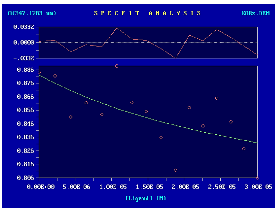
Slika 22. Odnos apsorbancije i povećanja koncentracije koridalina na valnoj duljini od 347 nm
