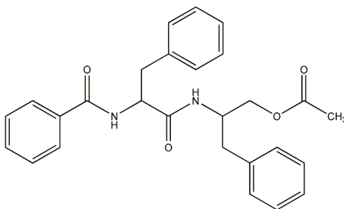
Slika 7. Aurantiamid acetat
