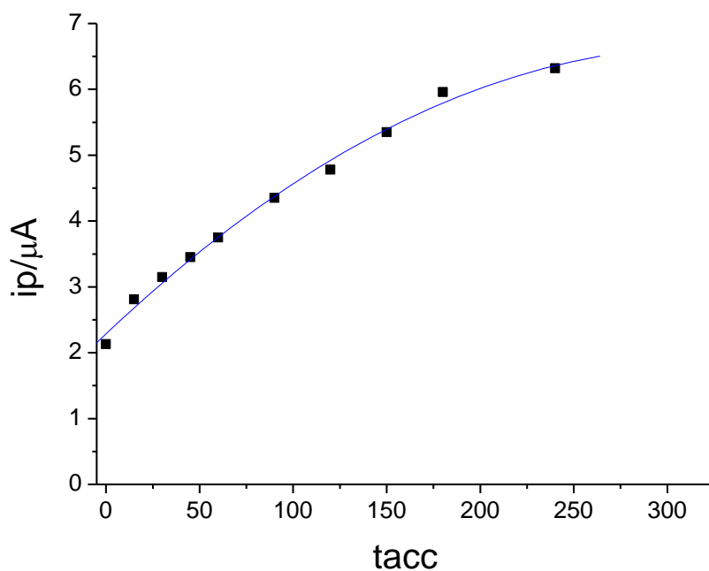
Slika 16. Grafički prikaz ovisnosti izmjenog strujnog vrha nepafenaka koncentracije 5 \times 10^{-6} M o vremenu akumulacije kod stripping SWV.
