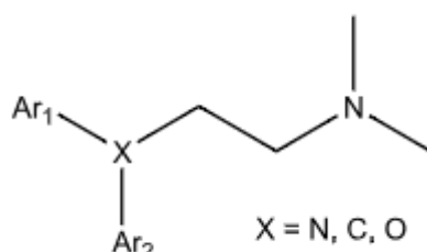
Slika 3. Opća formula H 1 -antihistaminika (prilagođeno prema Skidgel i sur., 2011)
