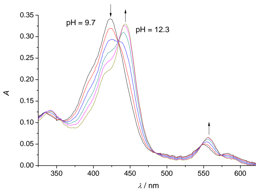
Slika 4.26. Tipična titracija 4,6 \mu\text{M} otopine Mn(III)TE-2-PyP u prisutnosti 0,1 \text{ mM } [\text{Mo}(\text{CN})_8]^{3-} u 2 \text{ M NaClO}_4 standardnom 0,2 \text{ M} otopinom NaOH ( t = 25 \text{ }^\circ\text{C} , l = 1 \text{ cm} ). Vrijednost pH otopine mijenjana je od 9,7 do 12,3 (neki spektri nisu prikazani radi preglednosti). Spektri zabilježeni u području pH < 9,7 prikazani su na slici 4.55.
