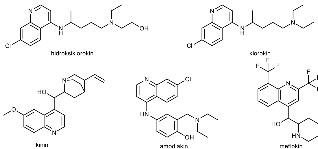
Slika 2. 4-Supstituirani kinolini
