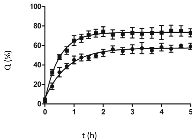
Slika 7. Profil oslobađanja melatonina iz lecitinsko-kitozanskih (●) i lecitinskih nanočestica (■). Ispitivanje je provedeno metodom dijalize uz acetatni pufer (pH 5,8) kao receptorski medij. Prikazane su srednje vrijednosti kumulativnog udjela oslobođenog melatonina ( Q ) \pm SD ( n = 3 ).
