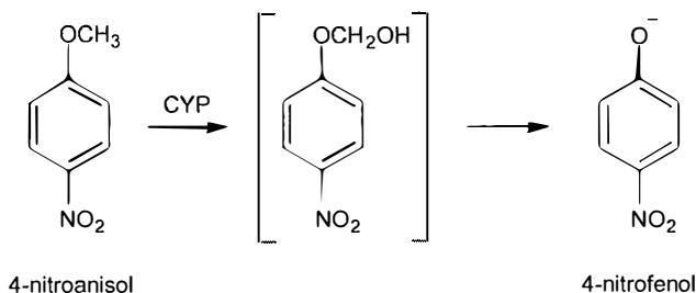
Slika 4. O-demetilacija 4-nitroanisolata
