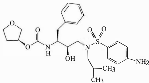
Amprenavir
