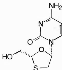
Lamivudin
