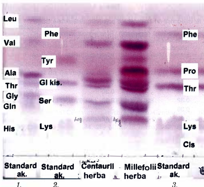
Slika 3.: Kromatogram aminokiselina zeleni kičice ( Centaurei herba ) i zeleni stolisnika ( Millefolii herba ).
