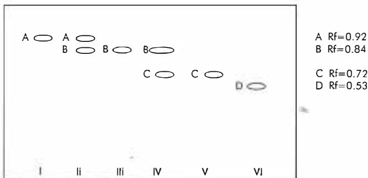
Sl. 2. TS-kromatogram flavonoidnih supstancija droge Flores bellidis izoliranih na stupcu \text{SiO}_2 Sustav otapala: etilacetat – mravlja kiselina – ledena octena kiselina – voda 100:11:11:27; Reagens za detekciju: Borna kiselina – oksalna kiselina 3:1 (6).
