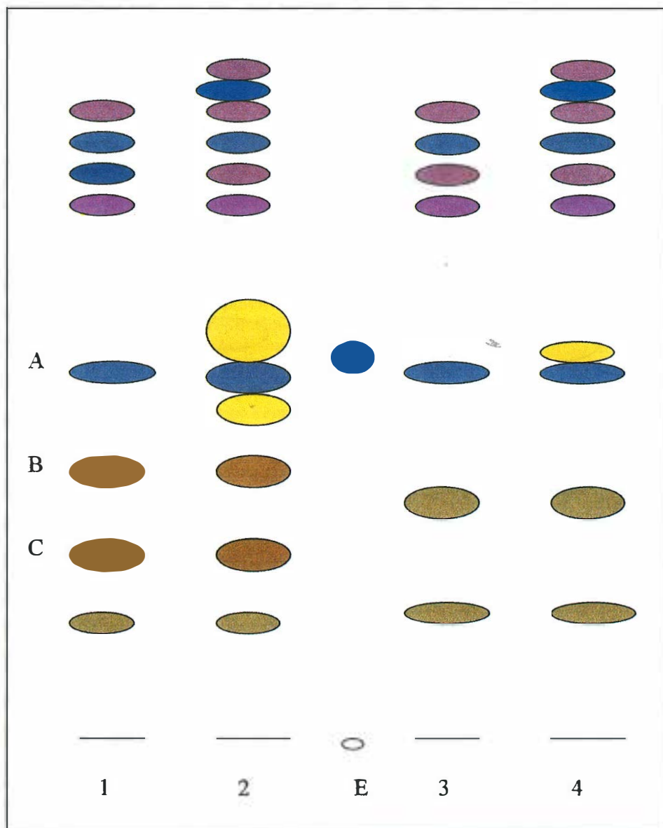
Slika 2. Kromatogram sastavnica vrsta E. repens i C. dactylon dobiven primjenom razvijaača kloroform-metanol-voda 64:50:10. Detekcija: klorsulfonska kiselina E =escin. 1,2,3,4, kao u Tablici 1.
