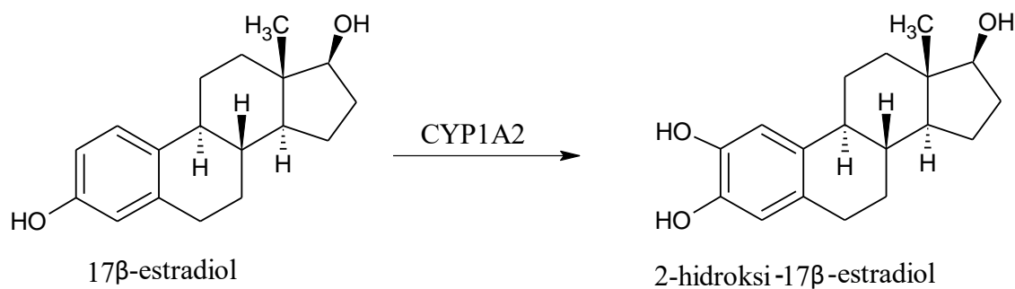
Slika 4. Reakcija hidroksilacije 17β-estradiola u položaju 2
