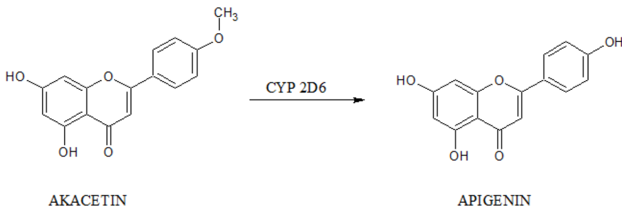
Slika 11. Demetilacija akacetina
