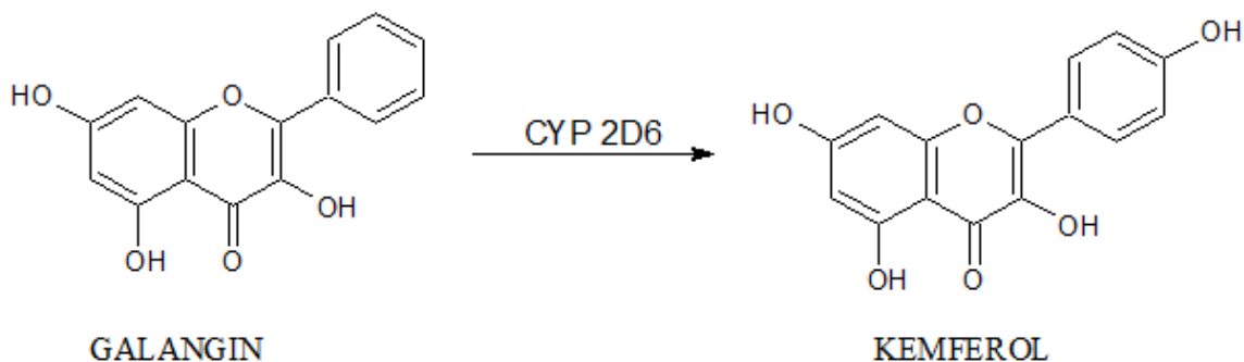
Slika 13. Hidroksilacija galangina
