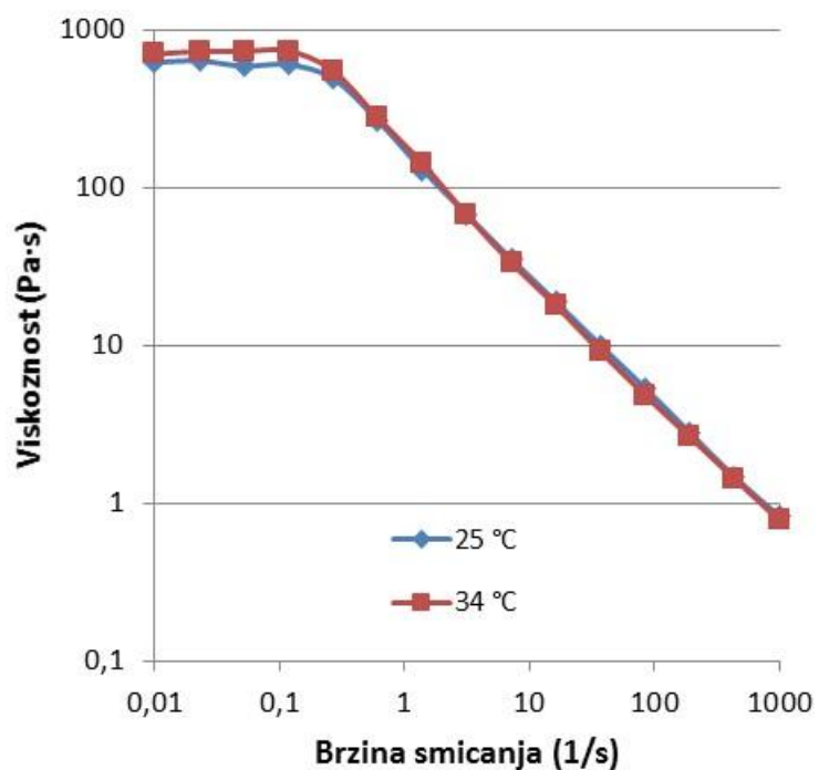
Slika 21. Viskoznost neutraliziranog kitozanskog gela na 25 i 34°C
