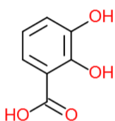
2,3-dihidroksibenzojeva kiselina
