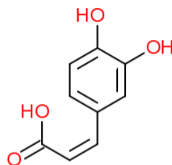
kavena kiselina
