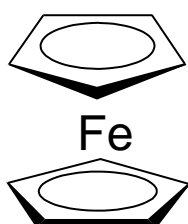
Slika 1. Strukturni prikaz molekule ferocena ( \text{FeC}_{10}\text{H}_{10} ).
