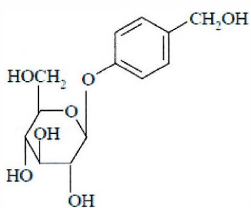
Gastrodin
