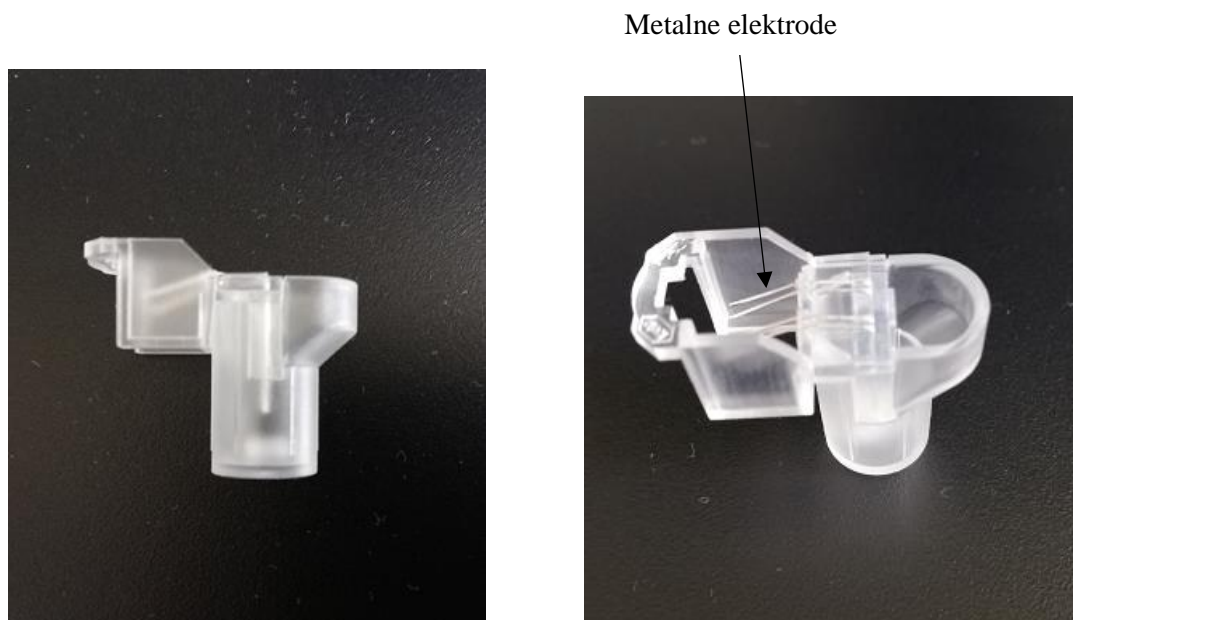
Slika 5. Ispitne kivete Multiplate uređaja (HZTM, Odjel za trombocitnu i leukocitnu dijagnostiku i hemostazu)
