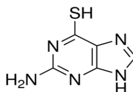
6-tiogvanin
