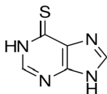
6-merkaptopurin
