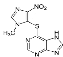
azatioprin
