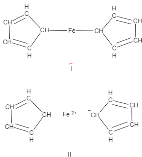
Slika 4. Prikaz struktura ferocena
