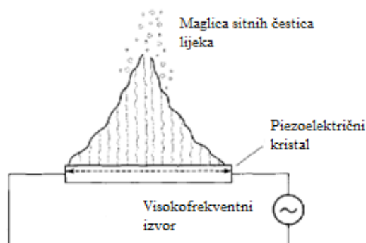
Slika 6. Shematski prikaz ultrazvučnog atomizatora (Atkins i sur., 1992.)
