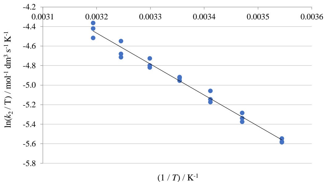
Slika 4.3.3. Eyringov prikaz ovisnosti \ln(k_2 / T) o 1 / T za reakciju katehina i DPPH• u smjesi otapala dioksan-voda (0,95:0,05 v/v). Reakcijska se smjesa sastoji od 0,003 \text{ mol dm}^{-3} katehina, 0,00005 \text{ mol dm}^{-3} DPPH• u smjesi otapala dioksan-voda (0,95:0,05 v/v). R^2 = 0,9819 . Podatci iz Tablice 4.3.1.
