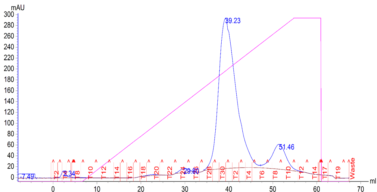
Slika 6. Kromatogram smjese nativnog transferina i \text{Fe}^{3+} u omjeru 1:1; primjer kromatograma visokog iskorištenja (Iskorištenje = 98,12 %)
