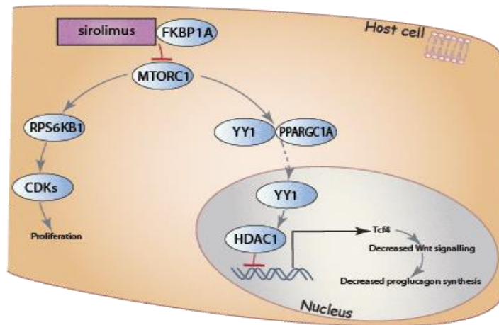
Slika 6: Put lijeka sirolimusa – farmakokinetika i farmakodinamika. Farmakokinetika - pojmovi: prijenosnik ABCB1; metaboliziranje putem CYP3A4 i CY3A5. Farmakodinamika: nakon ulaska u stanice, sirolimus tvori inhibitorski kompleks s imunofilinom FKBP-12 (kodiran genom FKBP1A ) koji cilja mTORC1, inhibirajući kaskadom reakcija posljedične učinke. Prikazan je i mehanizam zbog kojega djelovanje sirolimusa dovodi do određenih nuspojava: U citosolu se proteinski kompleks mTORC1 heterodimerizira s YY1 i PGC-1 \alpha da bi stvorio transkripcijski kompleks koji se podvrgava nuklearnoj translokaciji, kako bi aktivirao ekspresiju mitohondrijskog gena. Međutim, ovaj transkripcijski kompleks također može aktivirati histon-deacetilazu (engl. histone deacetylase , HDAC) u promotora TCF7L2 , gena koji kodira transkripcijski faktor Tcf4 koji olakšava ekspresiju ciljnih gena Wnt uzrokujući smanjenu sintezu proglukagona. Tako sirolimus pridonosi poremećajima homeostaze glukoze i dijabetesu nakon transplantacije (engl. new-onset diabetes after transplantation , NODAT). PharmGKB omogućuje upotrebu svojih podataka i sadržaja pod Creative Commons Attribution-ShareAlike 4.0 International License (8).
