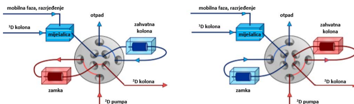
Slika 4. Shematski prikaz aktivne modulacije posredovane nepokretnom fazom - SPAM
