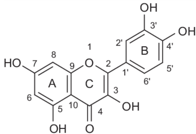
Slika 1.2.1.1. Struktura kvercetina
