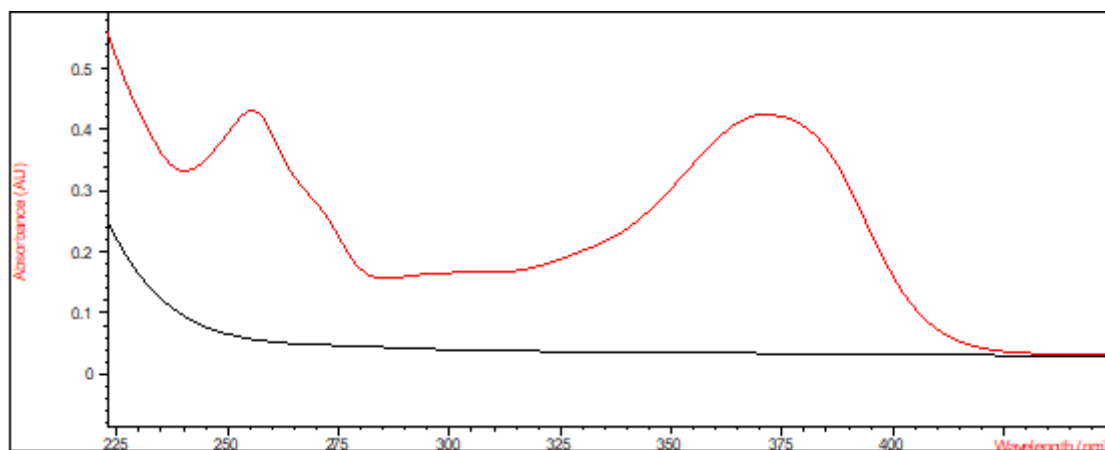
Slika 4.1.1. Spektar 2 \cdot 10^{-5} mol \text{dm}^{-3} otopine kvercetina u metanolu
