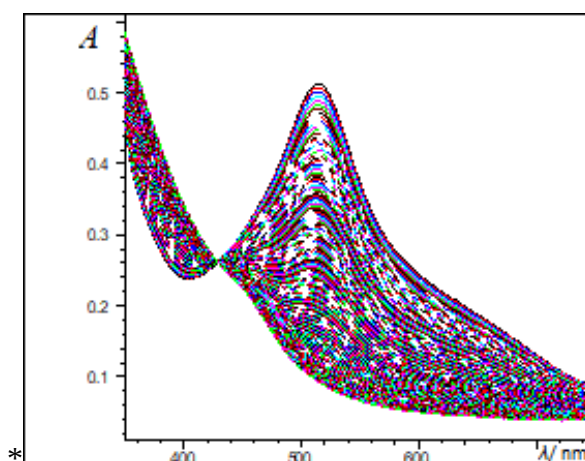
Slika 4.4.2. Spektralni profil reakcije katehina i DPPH• u otapalu metanolu pri koncentraciji katehina 2,5 \cdot 10^{-3} \text{ mol dm}^{-3} te koncentraciji DPPH• 5 \cdot 10^{-5} \text{ mol dm}^{-3}
