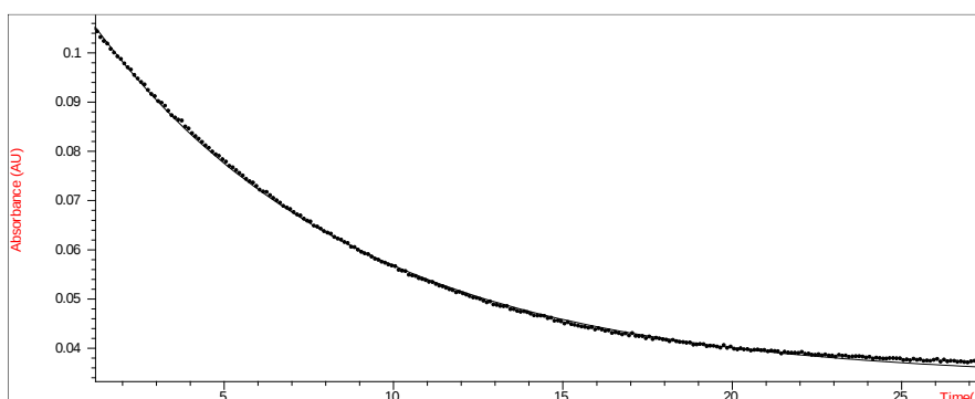
Slika 4.3.2. Ovisnost apsorbancije (A) DPPH• na 525 nm o vremenu (t) za reakciju kvercetina i DPPH• u metanolu pri koncentraciji kvercetina 2,5 \cdot 10^{-4} \text{ mol dm}^{-3} te koncentraciji DPPH• 3 \cdot 10^{-5} \text{ mol dm}^{-3} , pri temperaturi 25^\circ\text{C}
