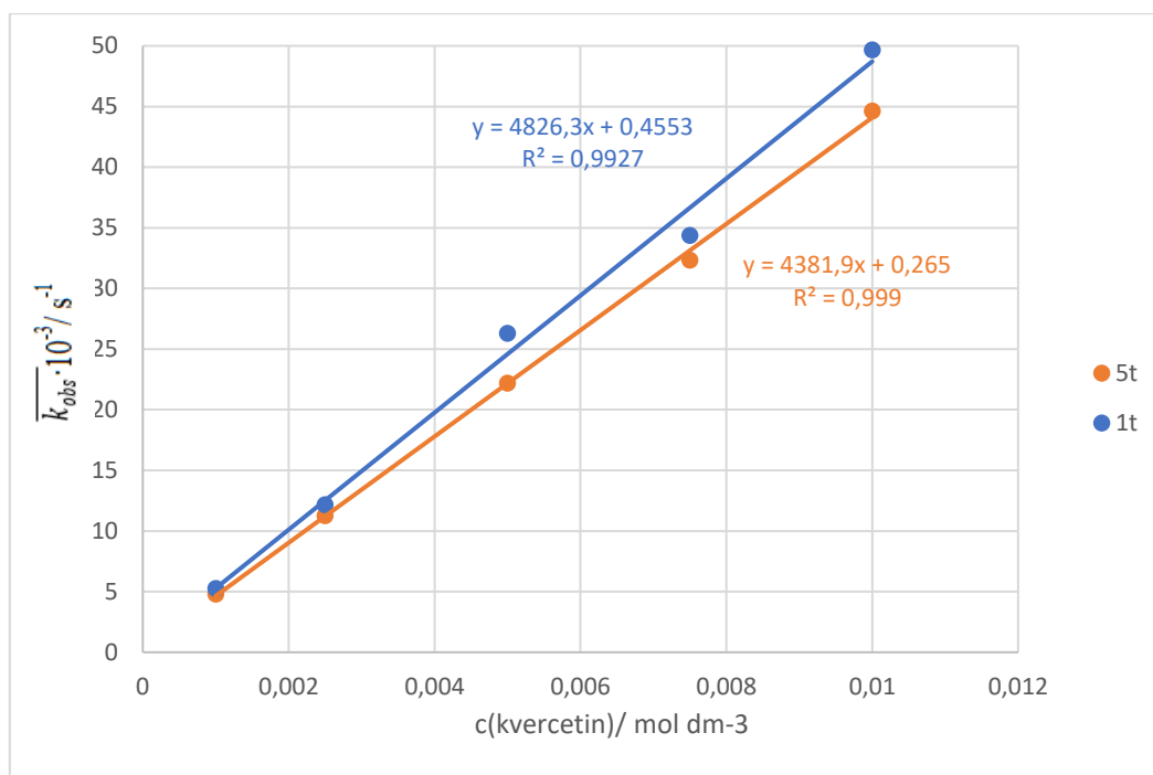
Slika 4.1.7. Prikaz ovisnosti konstante brzine ( \bar{k}_{\text{obs}} ) reakcije kvercetina i DPPH• u smjesi otapala dioksan-voda (0,99: 0,01 v/v) o koncentraciji kvercetina na 620 nm, izračunane iz intervala \sim 1 t_{1/2} (•) i \sim 5 t_{1/2} (•). Koncentracija DPPH• iznosi 5 \cdot 10^{-5} \text{ mol dm}^{-3} , pri temperaturi 25 °C. Podaci iz Tablice 4.1.3. te Tablice 4.1.4.
