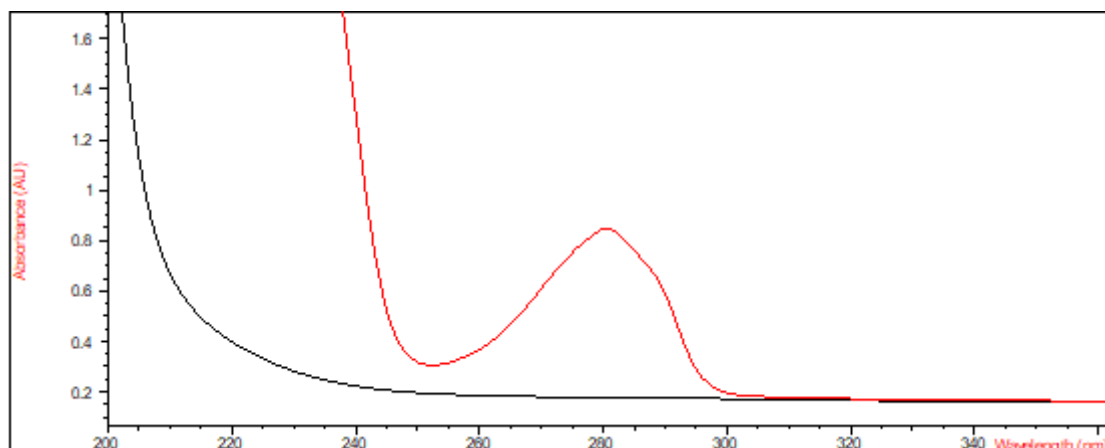
Slika 4.4.1. Spektar 2 \cdot 10^{-4} \text{ mol dm}^{-3} katehina u metanolu
