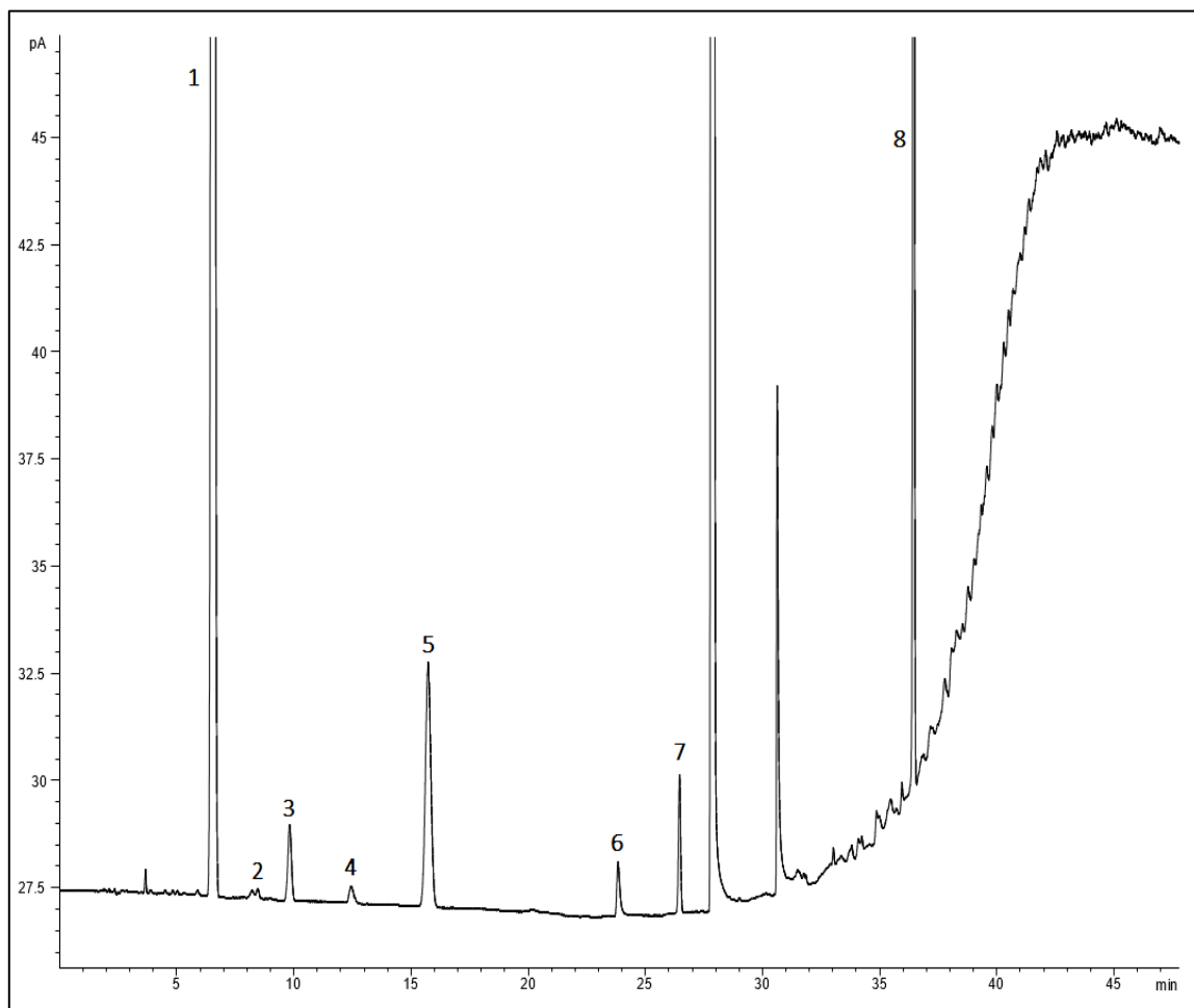
Slika 7. Kromatogram standardne otopine ostatnih otapala klase 2B pripremljene prema USP-ju
