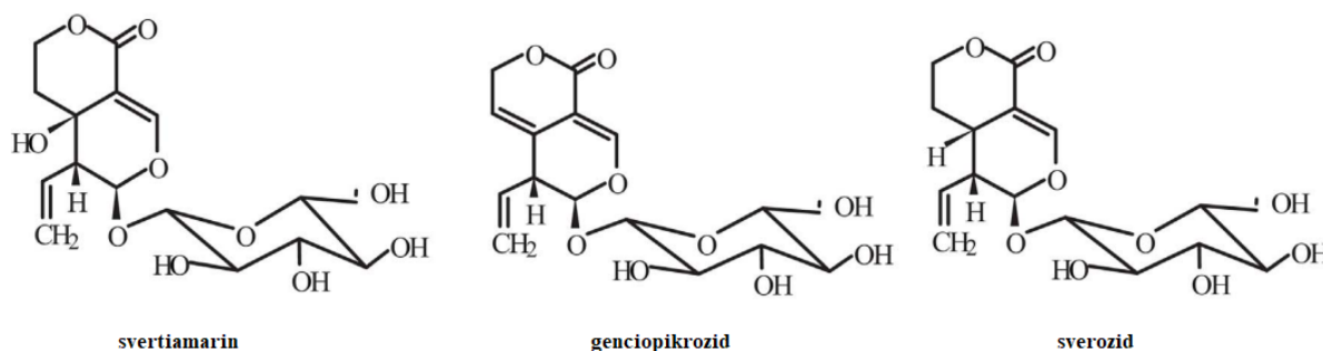
Slika 21. Kemijske strukture sekoiridoidnih glikozida prisutnih u Centaurium erythraea Rafn.
