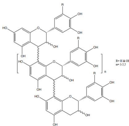
Slika 17. Kemijska struktura krofelemera (preuzeto i prilagođeno iz Frampton, 2013)
