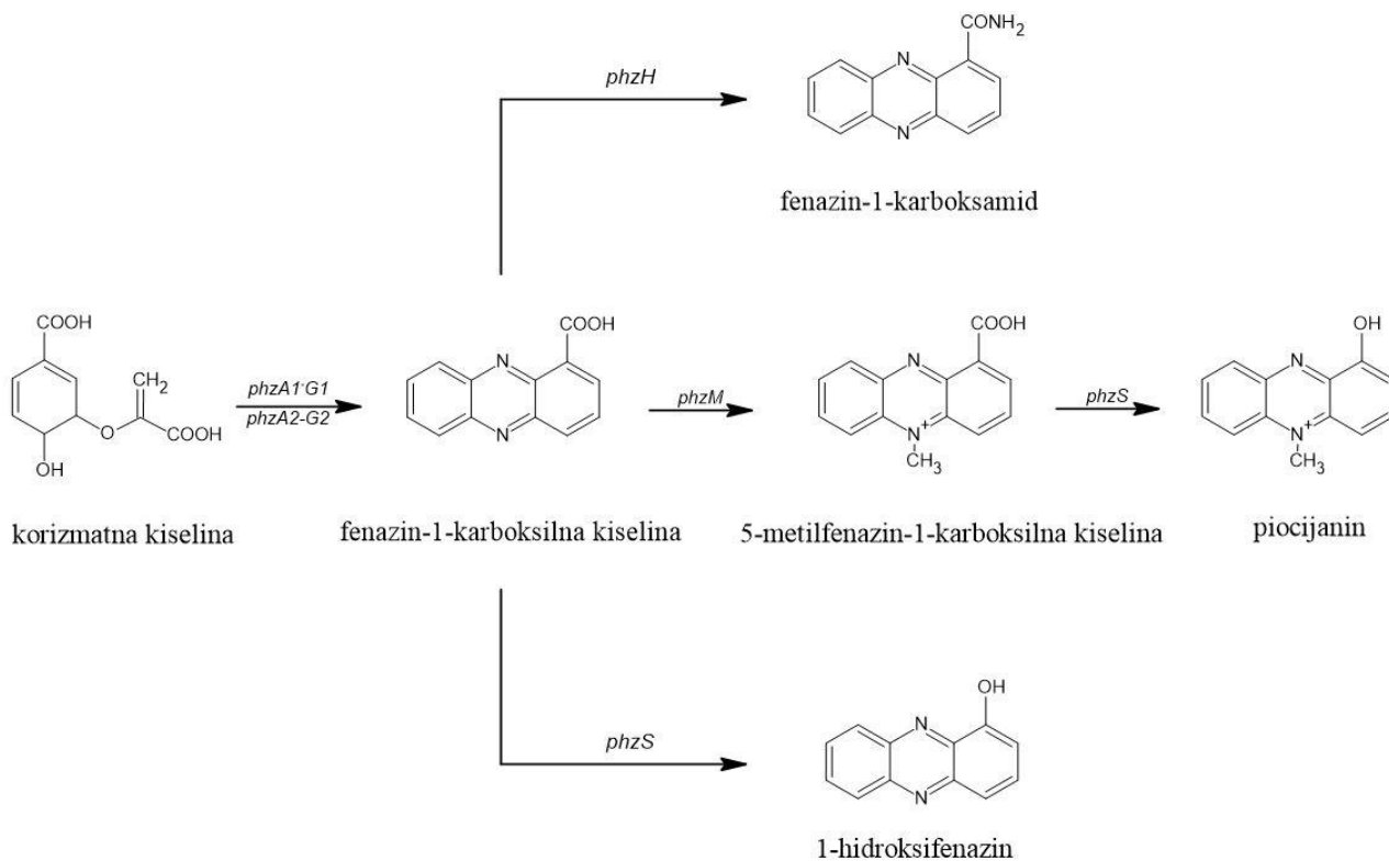
Slika 3. Sinteza piocjanina iz korizmatne kiseline.
