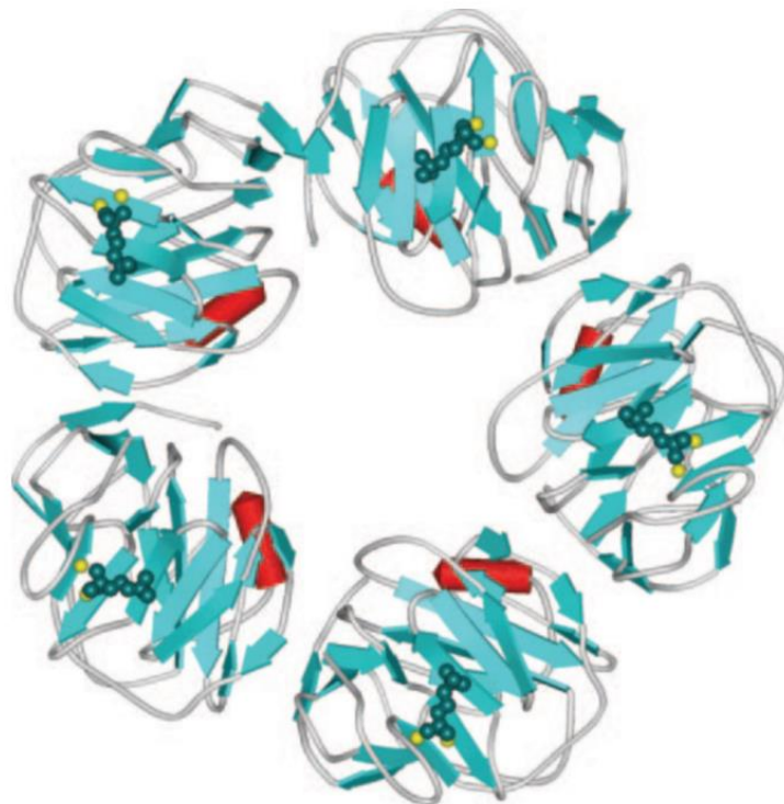
Slika 5: Kristalna struktura CRP-a u kompleksu s fosforilkolinom (preuzeto iz Black i sur. (2004) uz dopuštenje izdavača).
