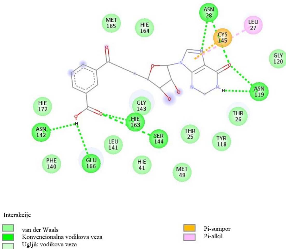
Slika 8. 2D prikaz broja i vrsta interakcija između furalozina i aminokiselinskih ostataka u aktivnom mjestu enzima (izrađeno pomoću programa Discovery Studio 2021).
