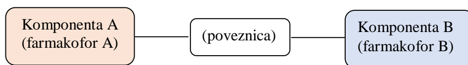
Slika 1. Pojednostavljeni prikaz hibridnih lijekova
