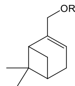
mirtenol mirtenil-acetat (R = acetat)
