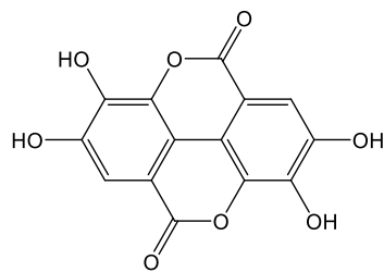
elagna kiselina
