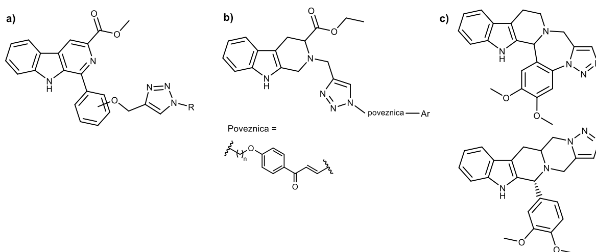
Slika 23. Triazolski derivati \beta -karbolina
