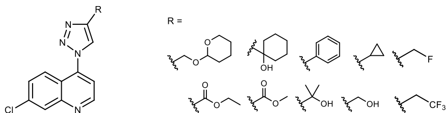
Slika 49. Hibridi 7-klorkinolina i triazola supstituiranih u položaju C-4
