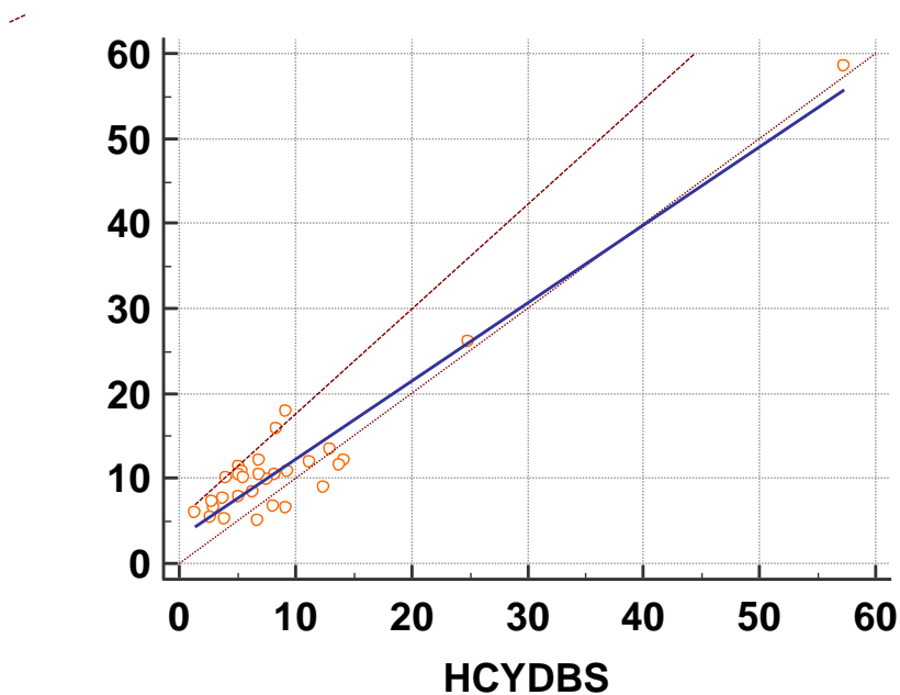
Slika 8: Prikaz Passing-Bablokove regresijske analize
