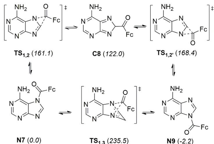
Shema 11a. Intramolekulski mehanizam (i) N7/N9 -transferrocenoiliranja adenina 2 : 1,2-pomak preko C8-ferrocenoiliranog intermedijera C8 (gornji dio sheme) i 1,3-sigmatropni pomak (donji dio sheme)
